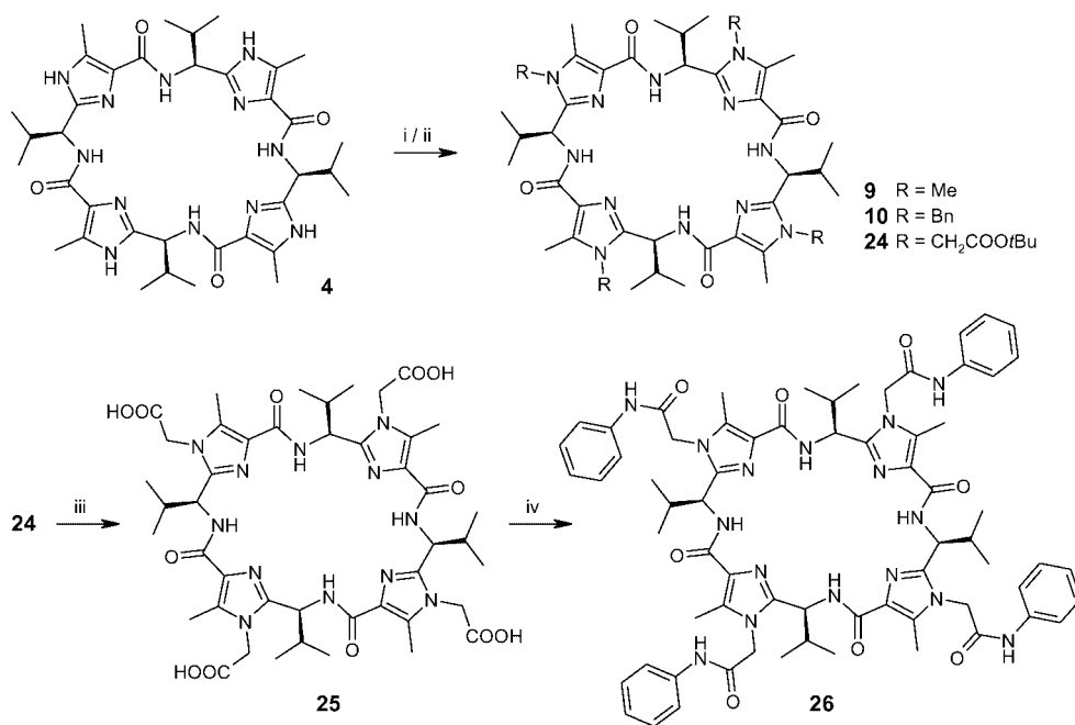
Scheme 6. i) RX, K 2 CO 3 , CH 3 CN, Δ. ii) RX, NaH, DMF, 0 °C → room temp. iii) TFA, DCM, quant. iv) DMC, aniline, Et 3 N, DCM, 0 °C → room temp., 44%.
